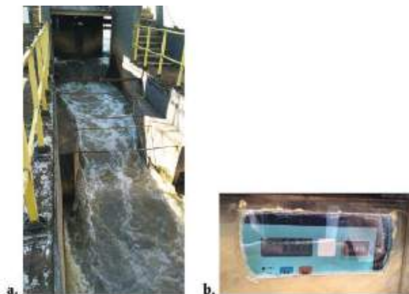
Figura 118 - ETE Franca - Setor 1 - Calha Parshall (a) e sensor de nível da Calha Parshall (b).
