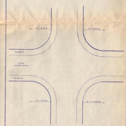
DETALHE DE CRUZAMENTO DAS RUAS ESCALA 1:300
